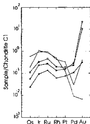
Figure 3.- Chondrite normalized PGE and Au of chromites. \square = Arroyo de La Cala, \star = Arroyo de Los Caballos, \Delta = Mina Baeza.
